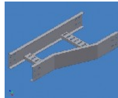
Thang cáp giảm bên phải Loại 1
